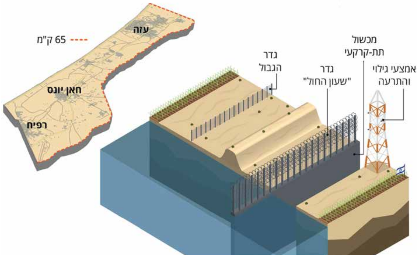
המכשול שבנייתו הושלמה ב-2021. מגננה נגד אימונים קרקעיים. דובר צה"ל
